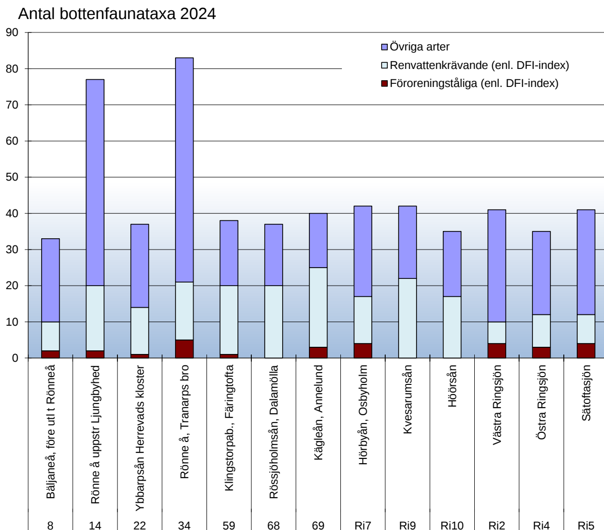
Figur 4. Antal taxa (hela stapeln) erhållna vid bottenfaunaundersökning inom Rönneåns vattensystem 2024, samt antal renvattenkrävande och smutsvattentålga arter enligt Dansk faunaindex (DFI). För förklaring till grupperna se metodik.
